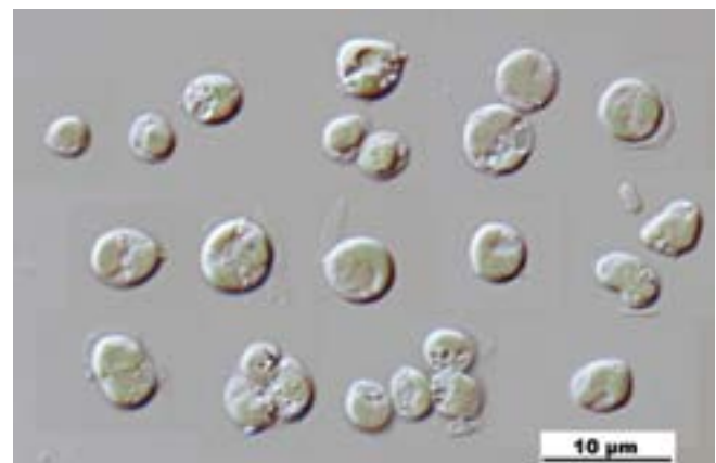
Fig. 5. Live algae Nanno. spp.
